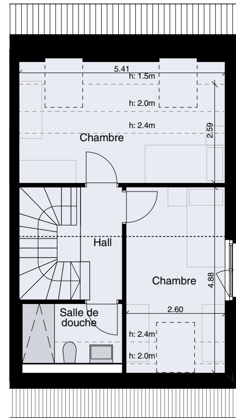
2 ème étage
