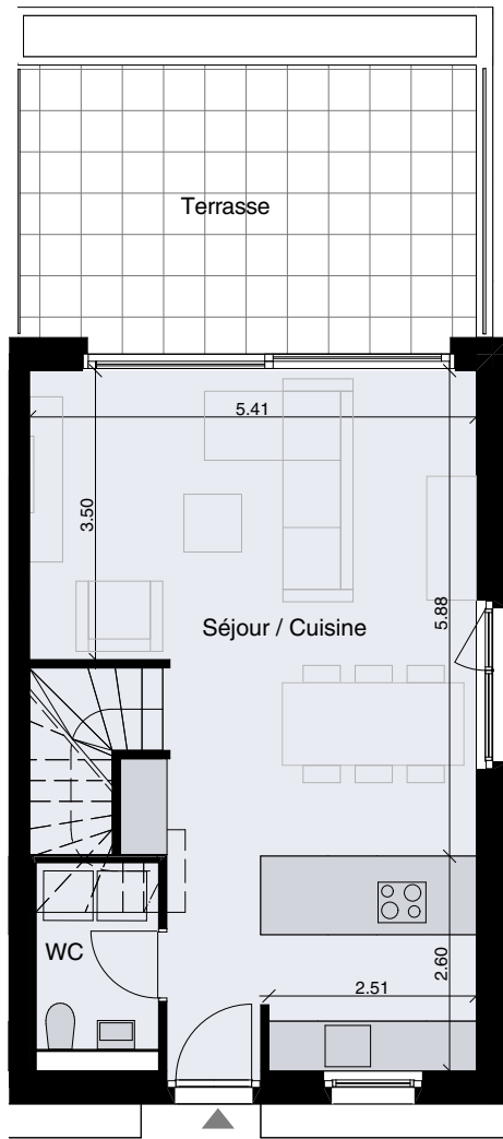
Rez-de-chaussée
